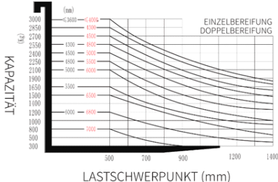
Hublastdiagramm
